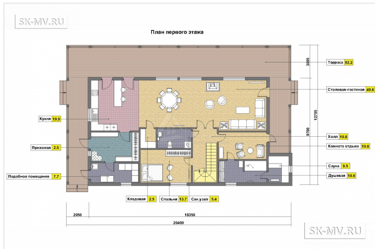
План первого этажа. Вариант 1
