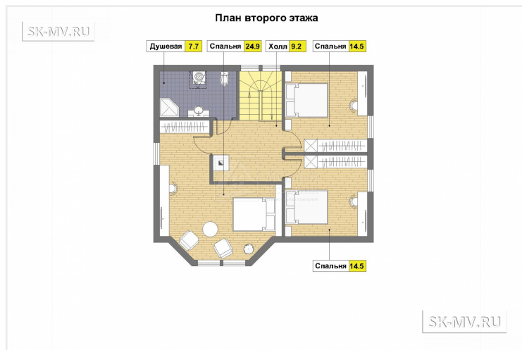
ПЛАН ВТОРОГО ЭТАЖА. Вариант 2
