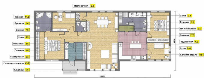
План первого этажа
